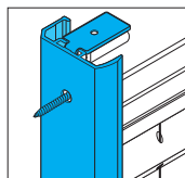
S3 Seitenführungsschienen U-Form 90°
